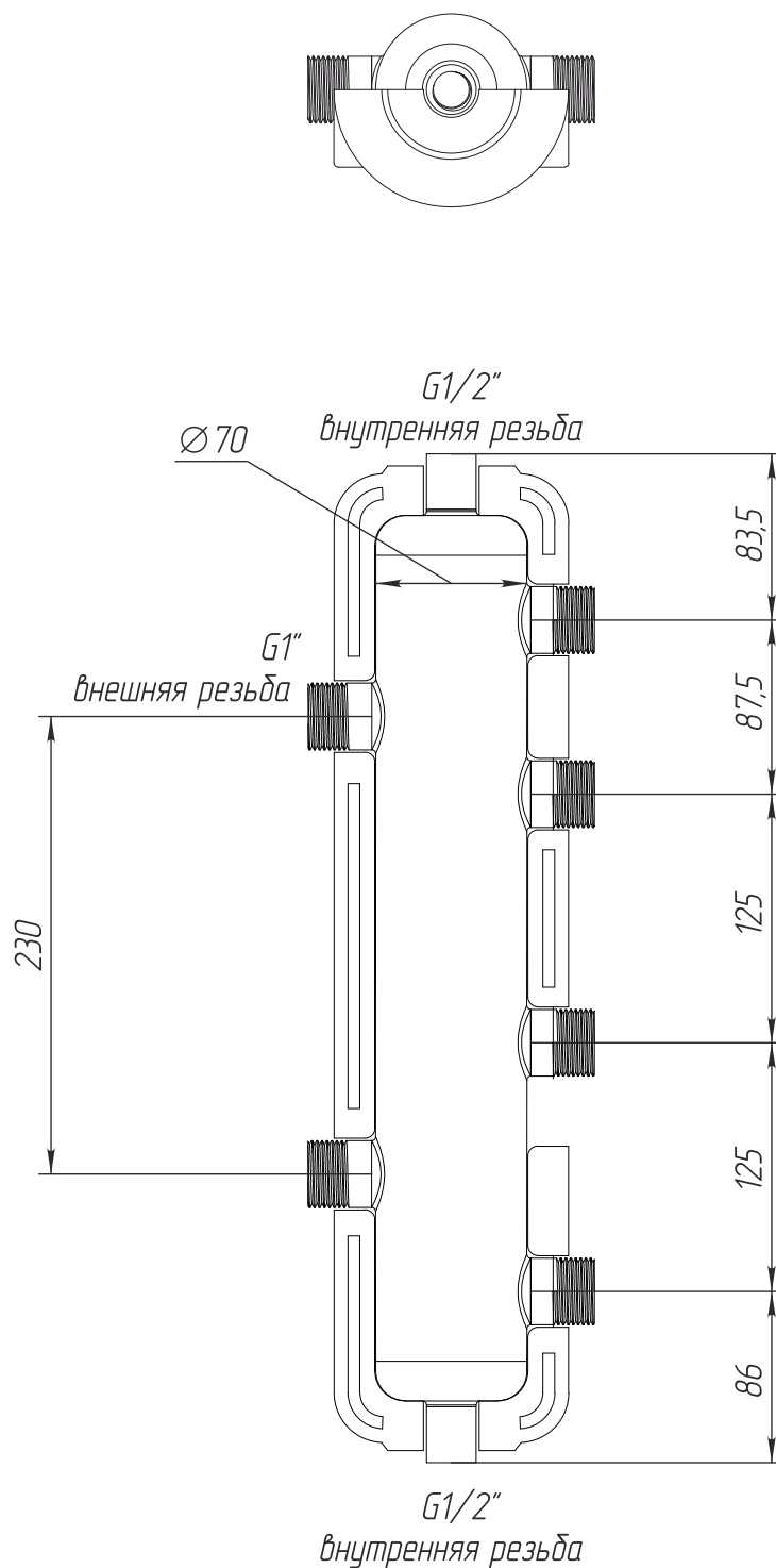
Рис.2 Гидроразделитель нержавеющий универсальный, 2 контура, до 60 кВт
