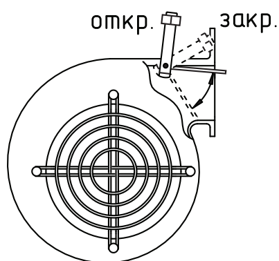
Рис.6 Вентилятор наддува
