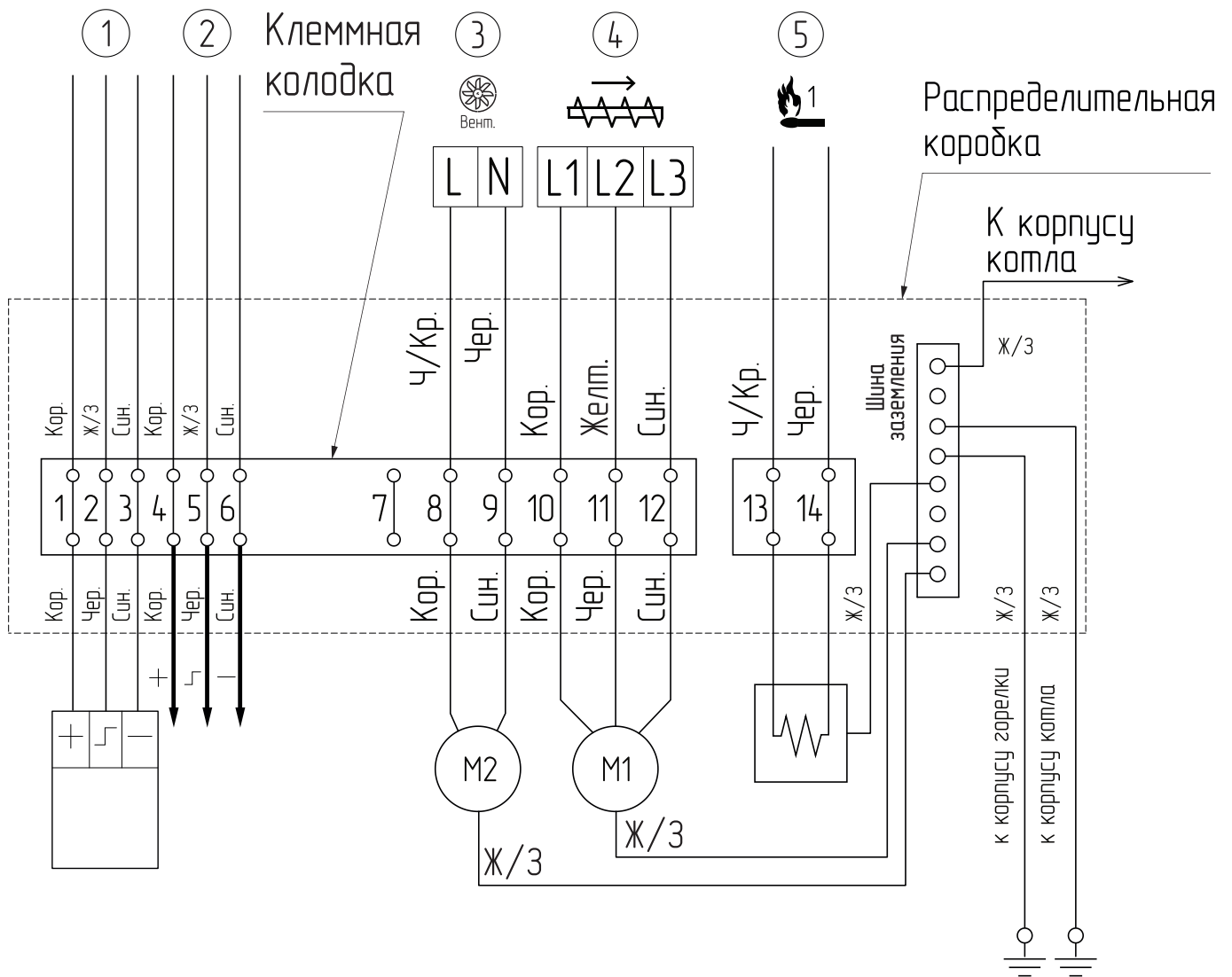
Рис.8 Схема распределительной коробки контроллеров ZOTA серии I-Line 224SFA для котлов ZOTA Pellet S
