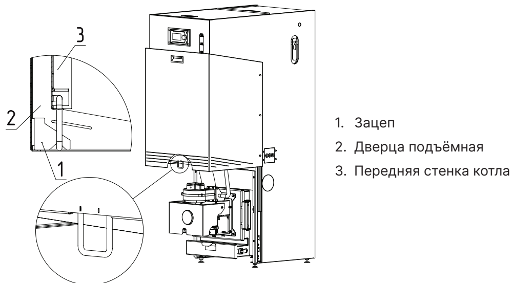
Рис.2 Зацеп двери котла ZOTA Pony
