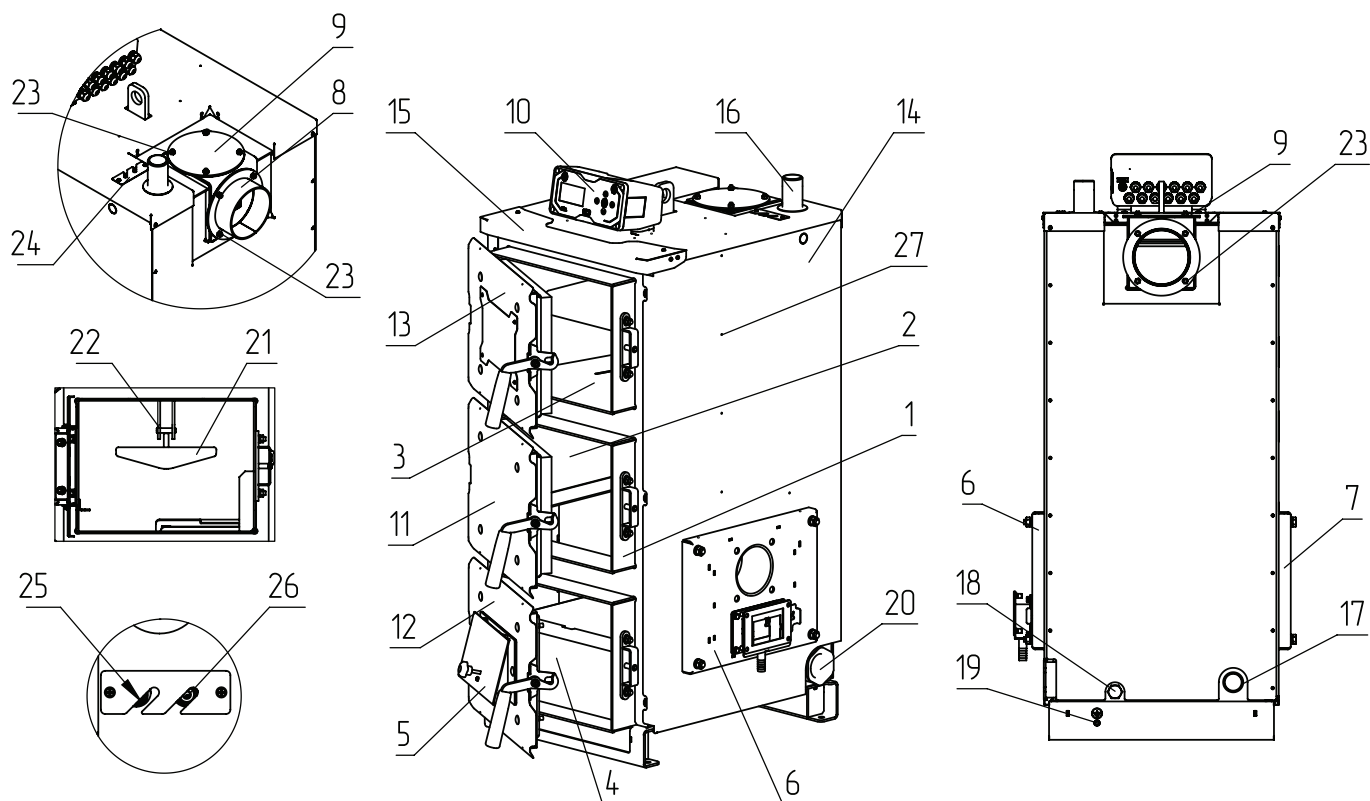
Рис.2 Конструкция теплообменника котла ZOTA Forta
