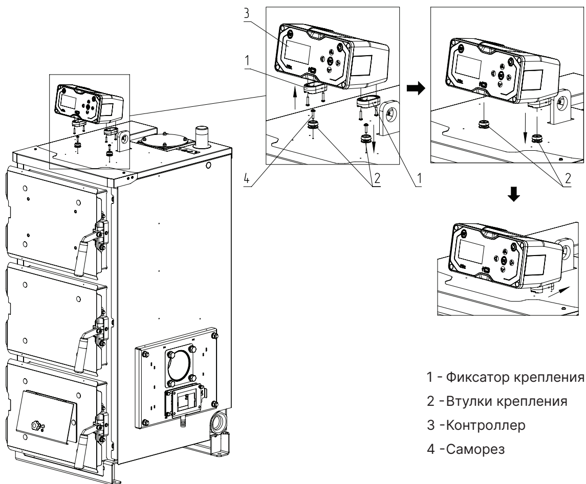
Рис.10 Монтаж контроллера
