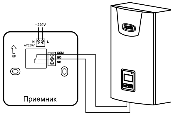
Рис.4 Схема подключения приемника.
