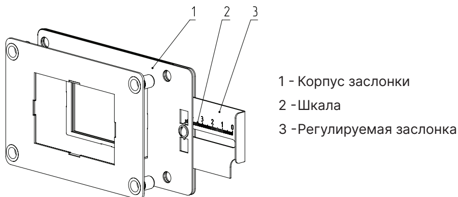
Рис.11 Заслонка вентилятора
