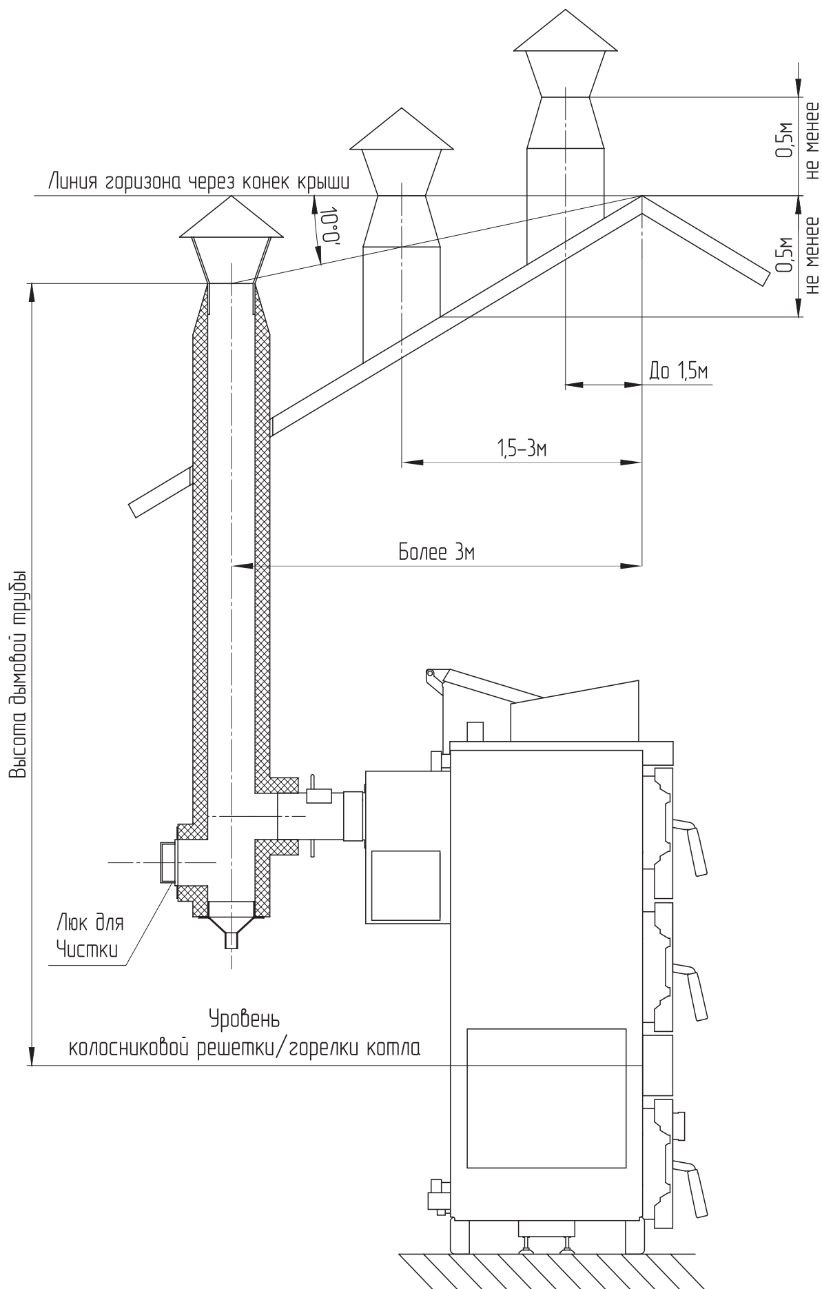
Рис.7 Варианты установки дымовой трубы
