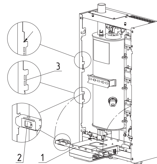
Рис.20 Откидывание кронштейна
