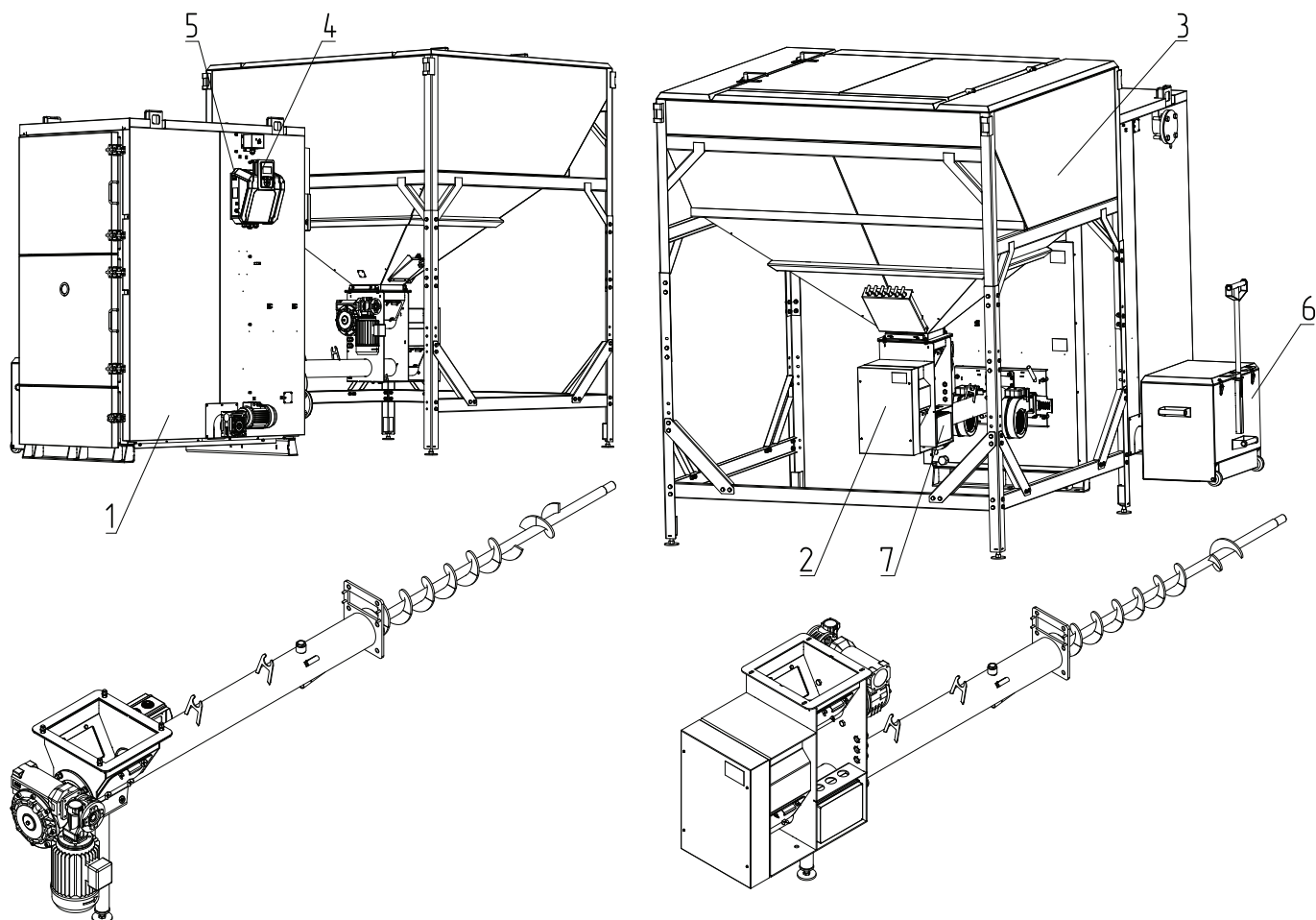
Одношнековый механизм подачи
