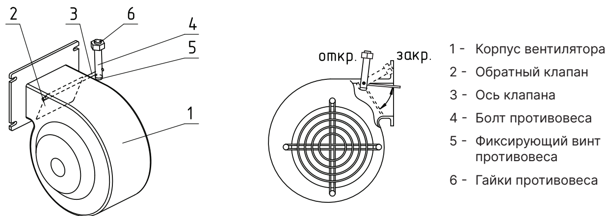
Рис.7 Вентилятор наддува
