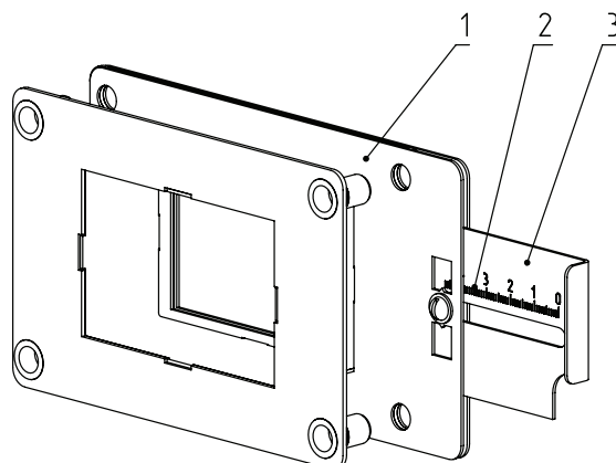
Рис.14 Заслонка вентилятора
