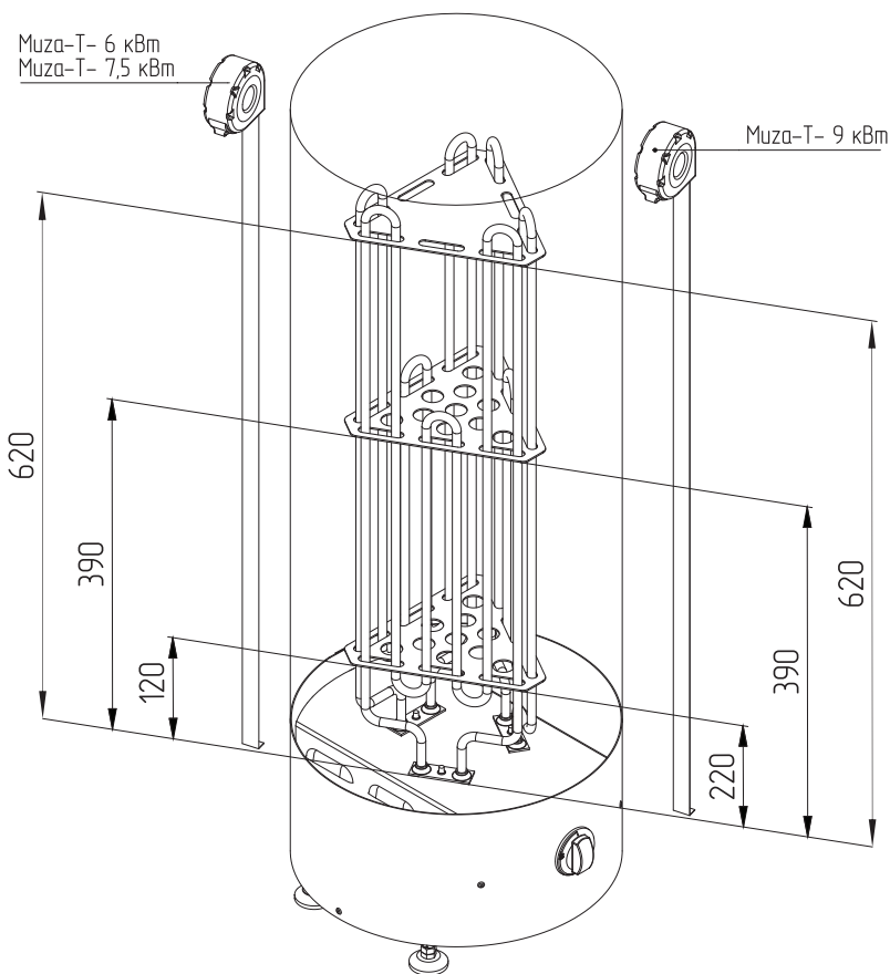
Рис.6 Расположение фиксаторов
