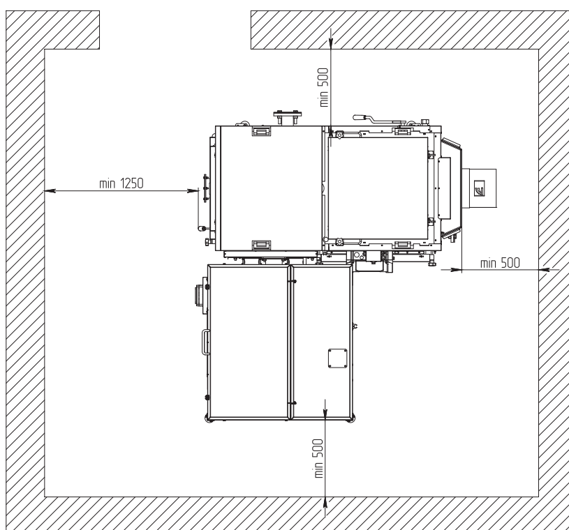
Рис.6 Расположение котла в помещении котельной
