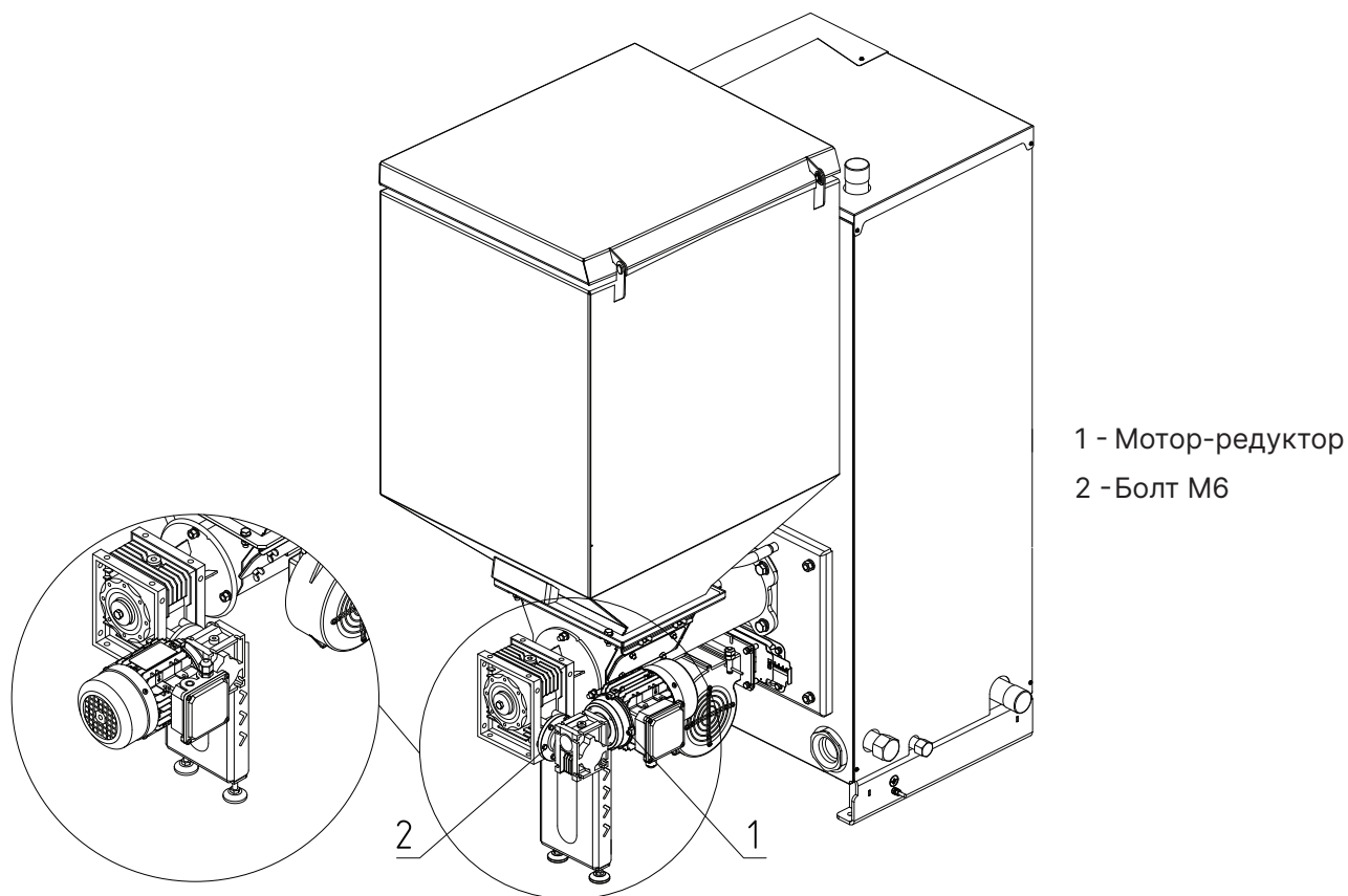
Рис.8 Изменение положение мотор-редуктора
