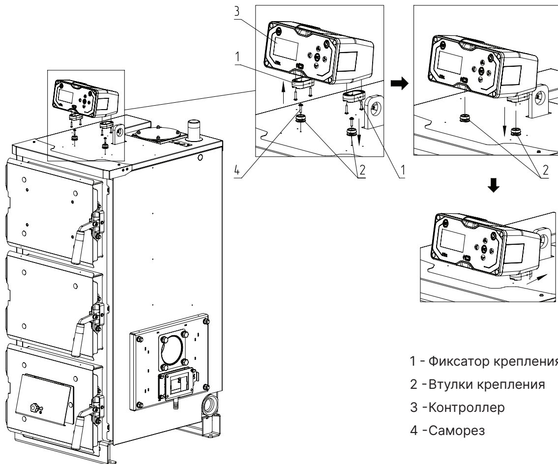
Рис.10 Монтаж контроллера
