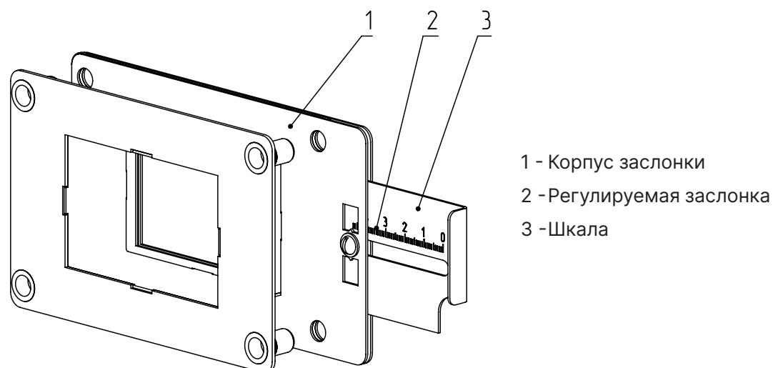
Рис.12 Заслонка вентилятора
