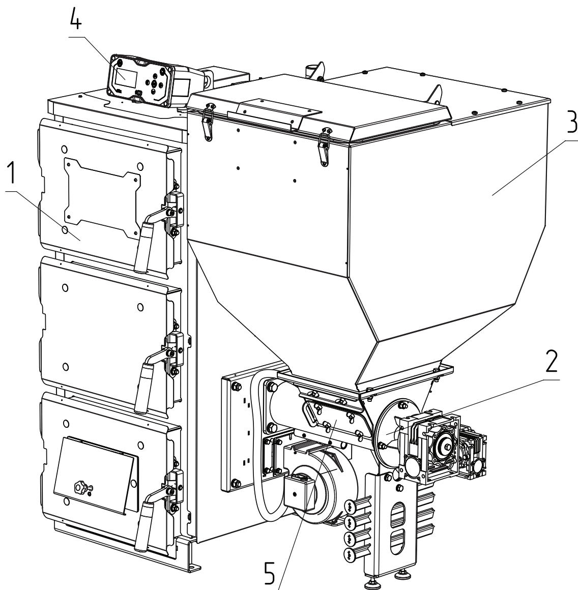
Рис.1 Конструкция котла ZOTA Forta
