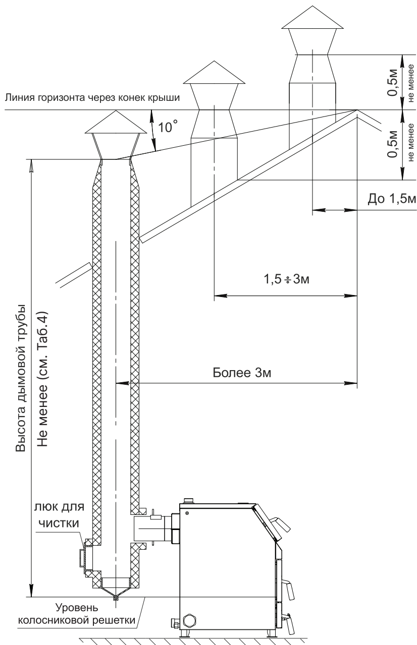
Рис.6 Варианты установки дымовой трубы
