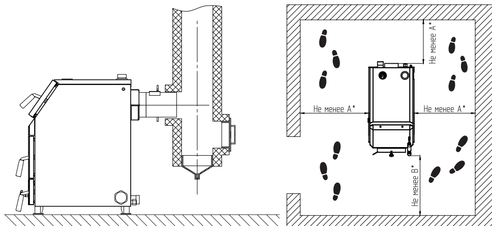
Рис.5 Расположение котла в помещении котельной
