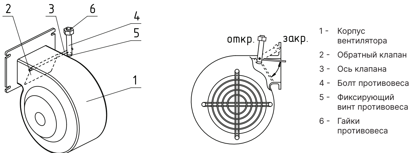
Рис.7 Вентилятор наддува
