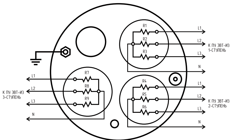
Б. Схема подключения к панели управления ПУ ЭВТ-ИЗ для котлов ZOTA Econom 18-48 кВт
