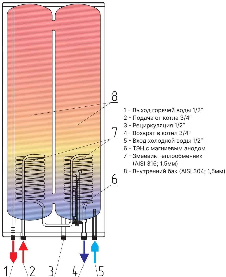
Рис.2 Внутреннее устройство водонагревателя
