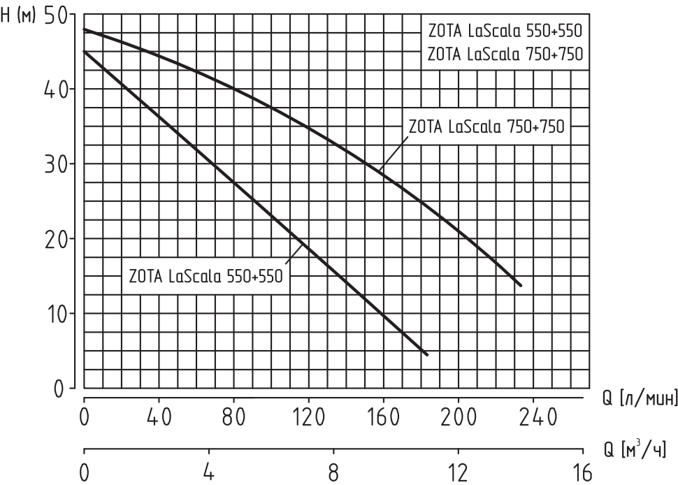
Рис.10 Диаграммы напорно-расходных характеристик насосных станций
