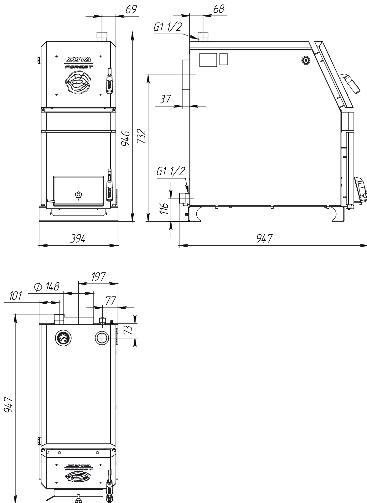
Рис.3 Монтажные размеры твердотопливного котла ZOTA Forest 31
