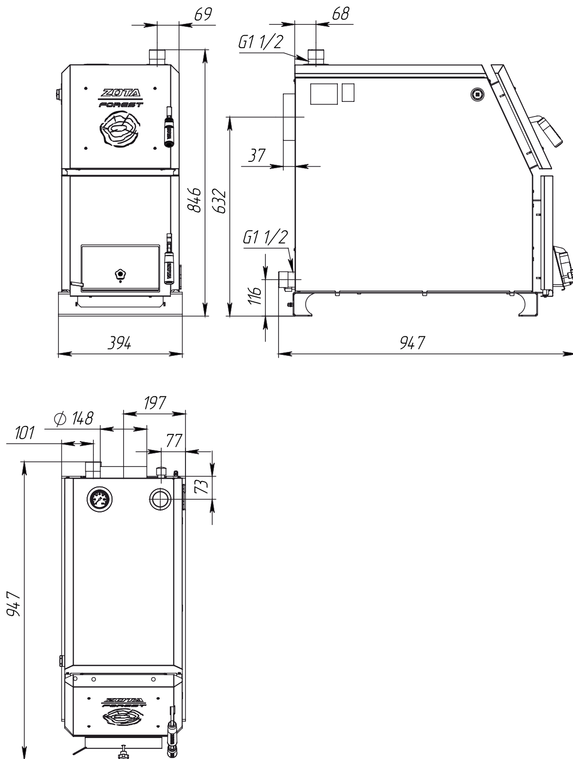
Рис.2 Монтажные размеры твердотопливного котла ZOTA Forest 21
