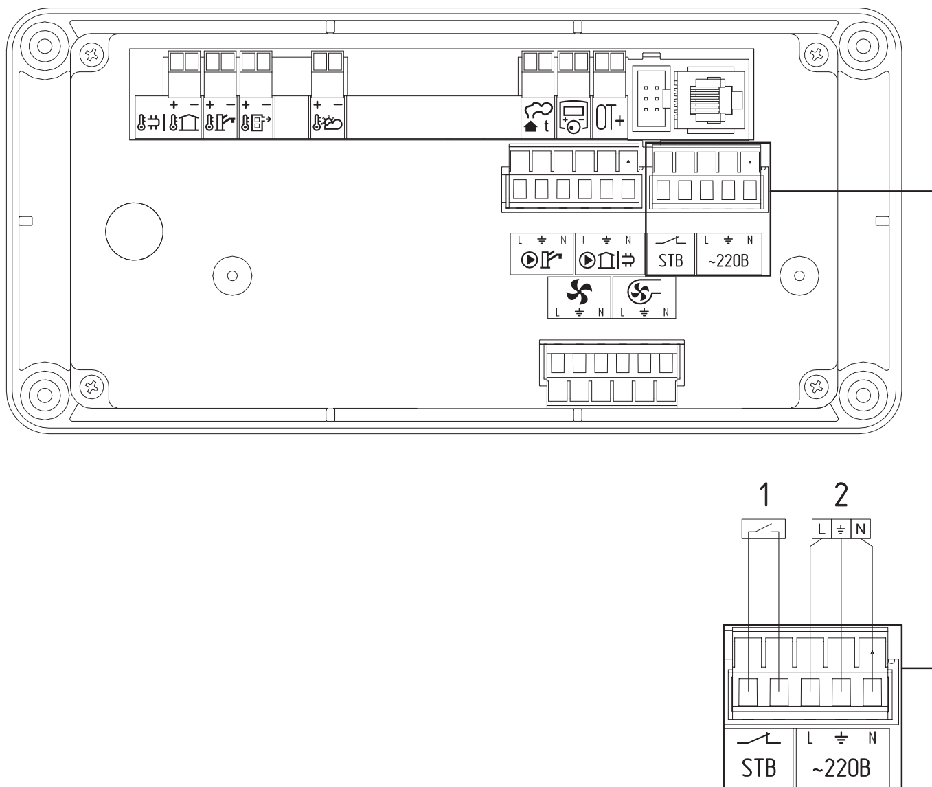
Рис. 6 Схема подключения термоограничителя и шнура питания к контроллеру ZOTA серии C-Line 200SF
