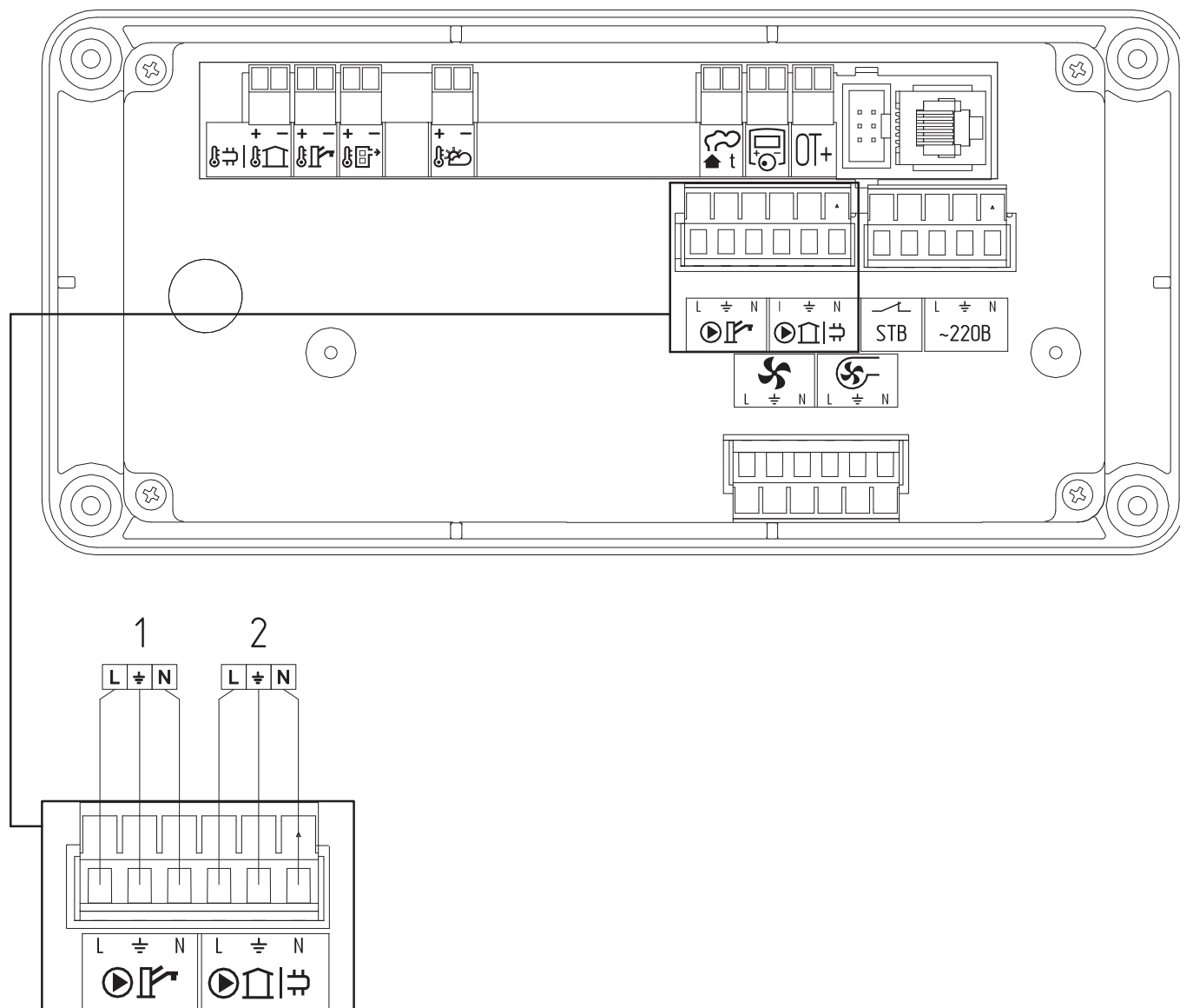
Рис. 8 Схема подключения циркуляционных насосов
