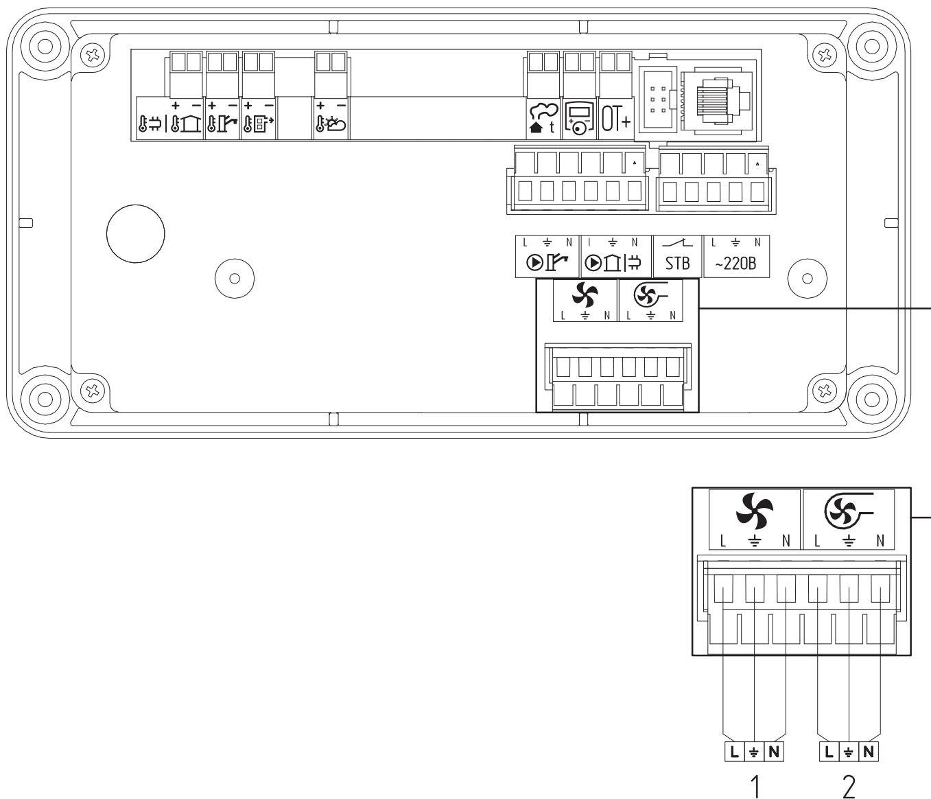
Рис. 9 Схема подключения механизма подачи топлива, вентиляторов наддува, дымососа
