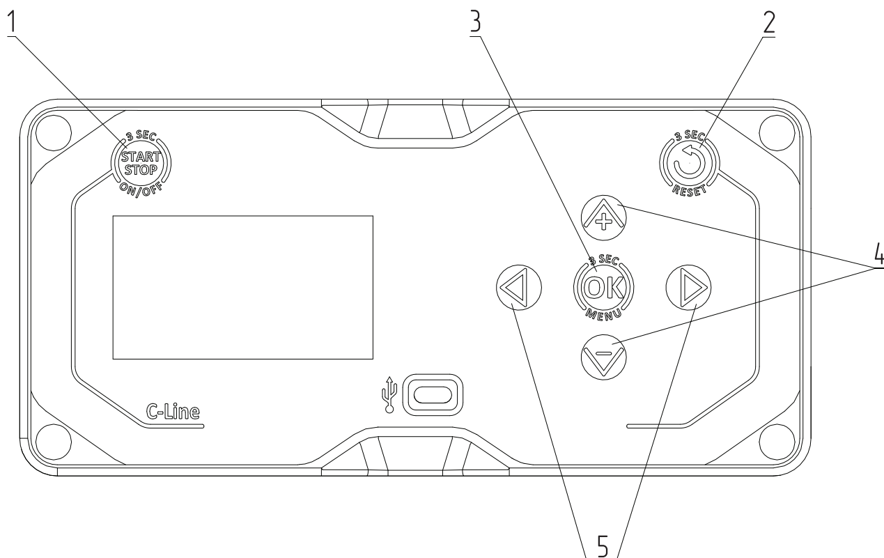
Рис. 10 Функциональные клавиши контроллеров ZOTA серии C-Line 200SFA
