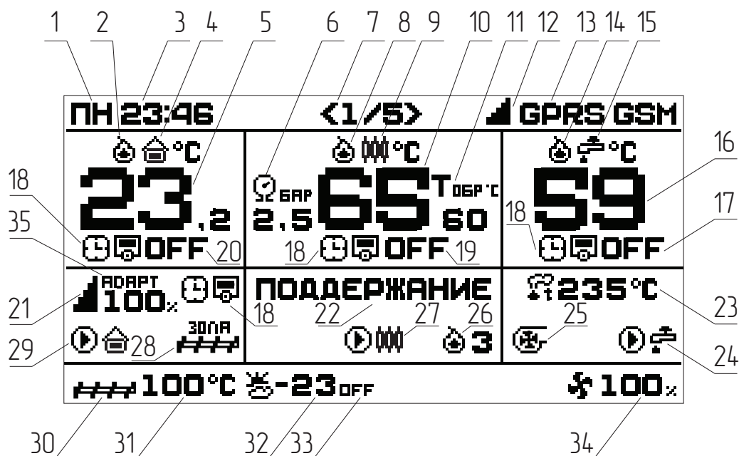
Рис. 11 Дисплей контроллера ZOTA серии C-Line 200SFA
